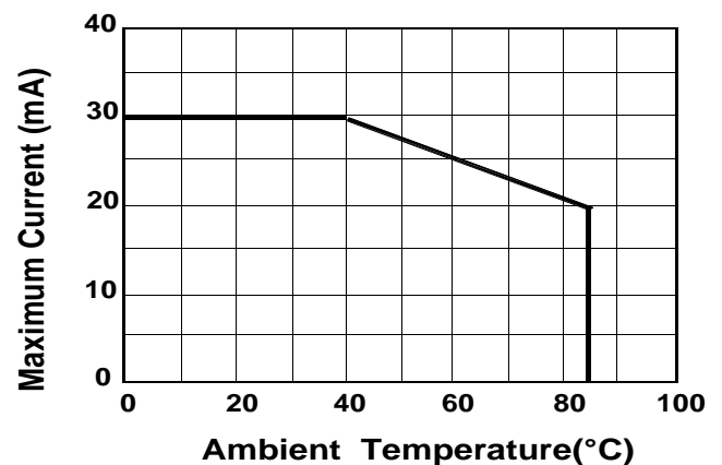
8).Thermal Design
