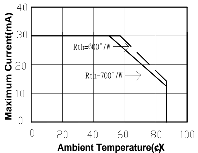
8). Thermal Design
